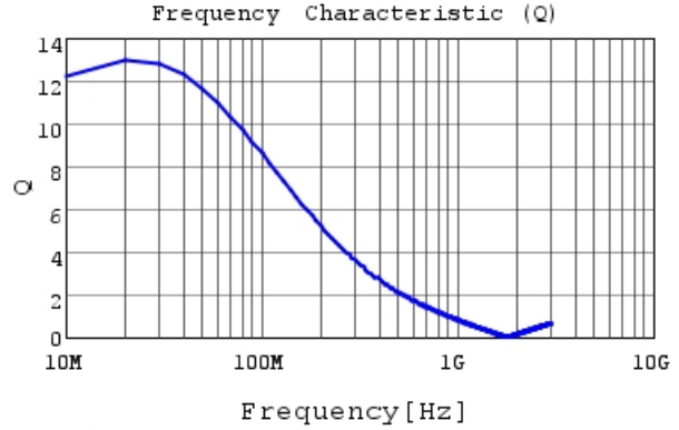
LQW18CNR16J00 Q
