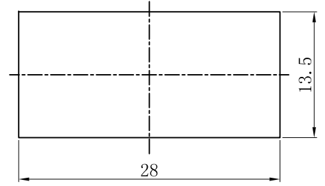
安装面板尺寸 PANEL CUT-OUT
