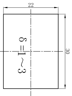
安装面板尺寸 PANEL CUT-OUT
