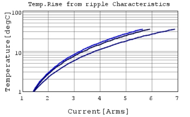
GCM32ER71E106KA57 Temp.rise — 80kHz
