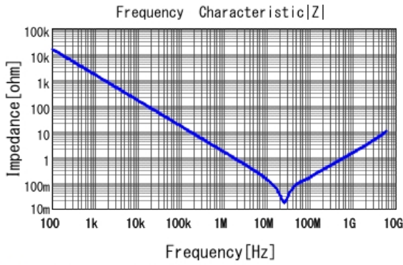
■ GRM155C71H104KE19 |Z| DCOV, 25degC
