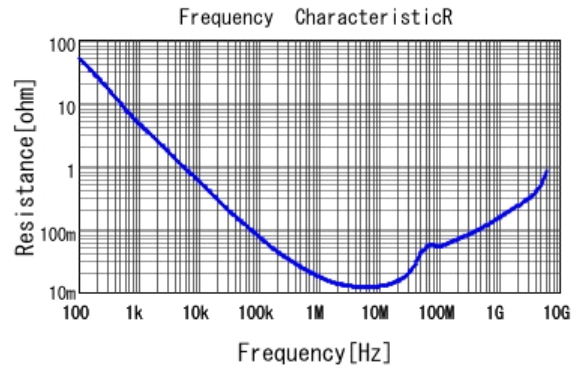
■ GRM155C71H104KE19 R DCOV, 25degC
