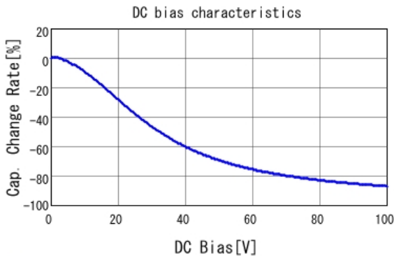
■ GCJ32DC72A475KE01 C-DC bias capchange, 25.0degC, AC1.
