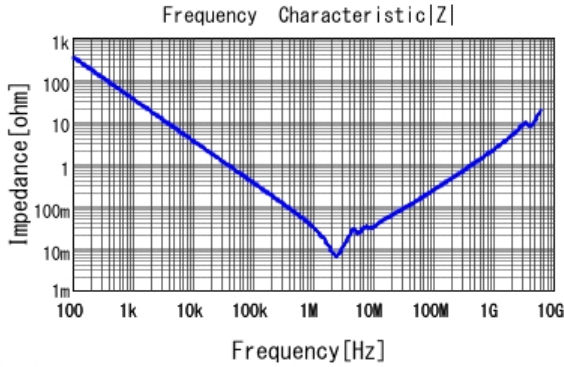
■ GCJ32DC72A475KE01 |Z| DC0V, 25degC
