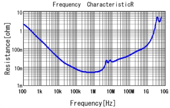
■ GCJ32DC72A475KE01 R DC0V, 25degC
